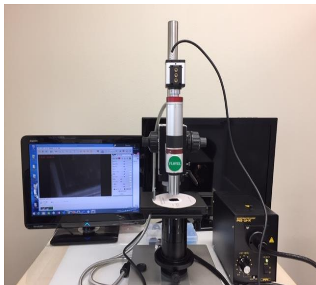
ウェハー 透過による検査
